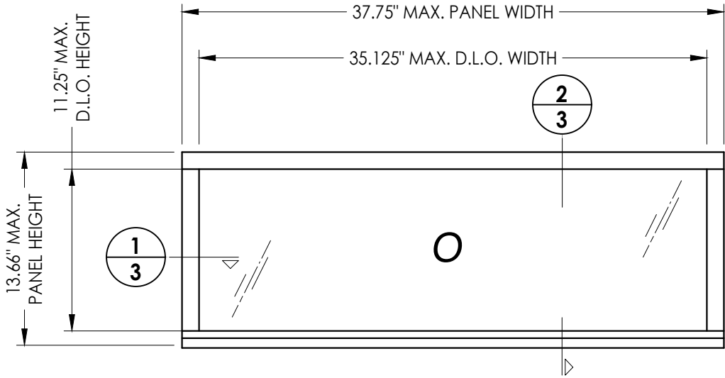
70 Transom
